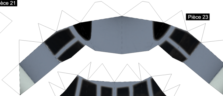
Pièce 21
